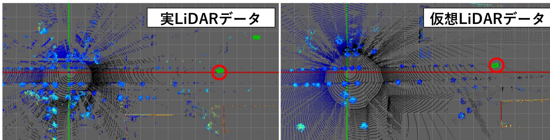
物体検出例 (対象までの距離: 約110m, 赤丸: 認識対象, 緑矩形: 検出結果)
