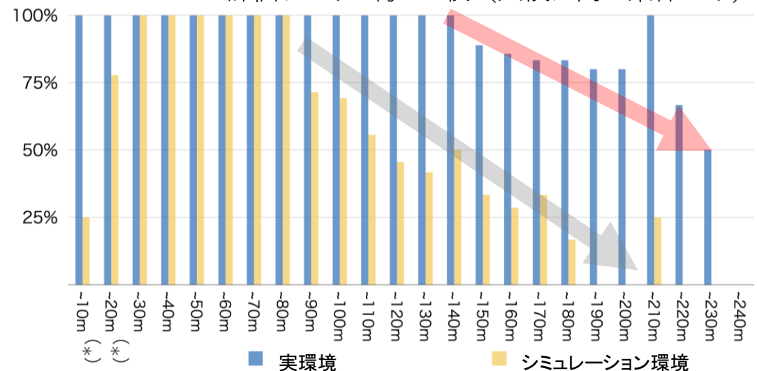
物体検出による精度比較 学習データ: 東京都臨海部データセット 21,401枚 評価データ: 約200枚 (天候は同一条件のみ)
